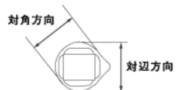
図7. 剣先の直径測定例(完成品)
